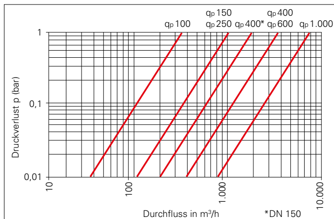
Druckverlustkurve
